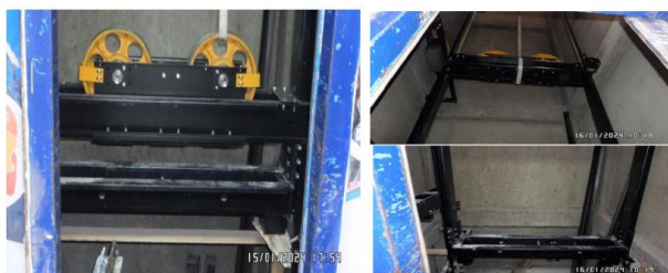
Ensamble de marco de cabina y plataforma (piso) ascensor No. 4
