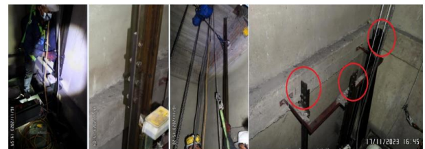
Desmante de sistema de rieles guía y soportes de ascensor No. 4
