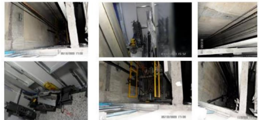
Desensamble de soportes y rieles guía y accesorios , ascensor No. 1
