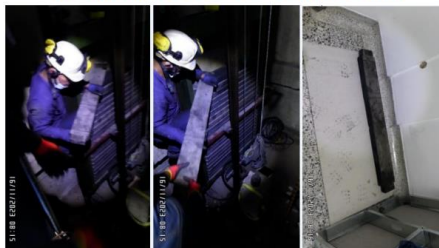
Desmantelamiento del sistema de contrapeso ascensor No. 4
